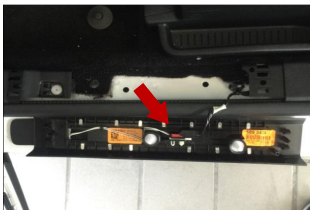
拆内饰件 拆迎宾踏板时注意避免损坏原车灯线(箭头)
